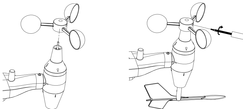
Obr 5: Nákras instalace pohárků na měření rychlost větru
