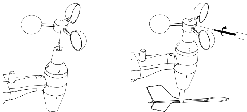
Obr 5: Nákras inštalácie pohárikov na meranie rýchlosti vetra
