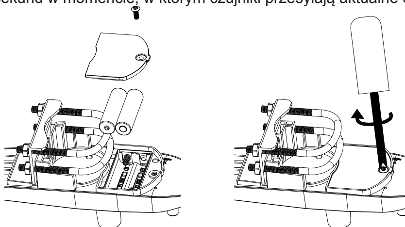
Rycina 7: sposób instalacji baterii
